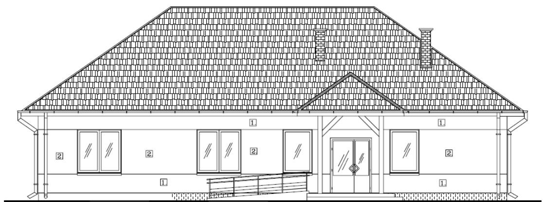
ELEWACJA FRONTOWA
